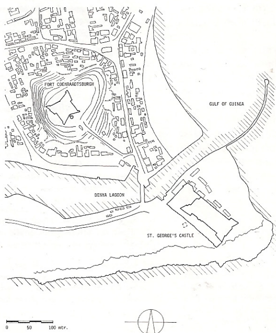
Afb. 1 Situatie van het kasteel St. George d'Elmina en fort Coenraadsburgh op de heuvel St. Jago (tekening auteurs).
